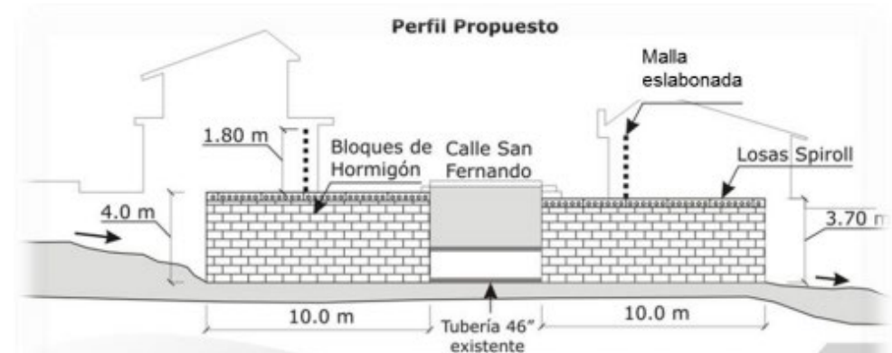
Propuesta de soluciones grises y jardines infiltrantes en los laterales. Tramo I.
