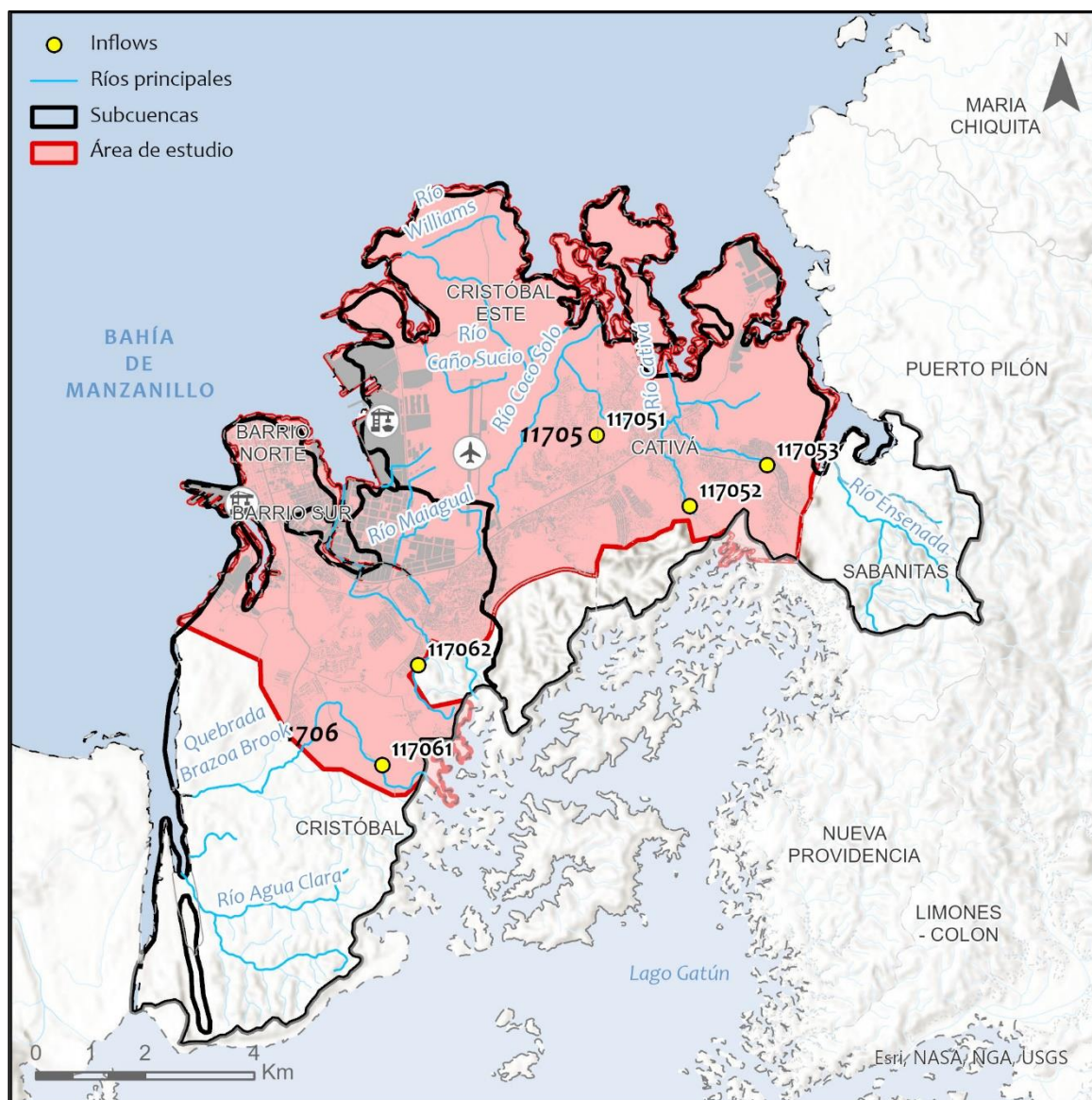
Figura 64. Puntos de entrada de caudales en el modelo hidráulico. Fuente: IHCantabria, 2024.
