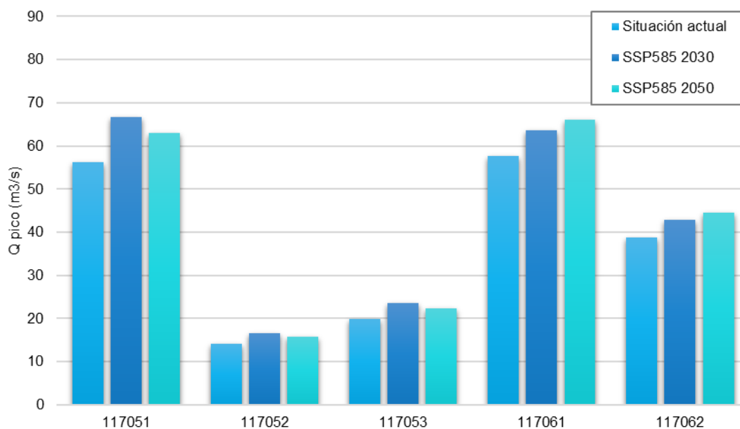
Figura 65. Caudales pico en los puntos de entrada de caudal en el modelo hidráulico para los eventos de periodo de retorno de 100 años en los diferentes escenarios climáticos. Fuente: IHCantabria, 2024.
