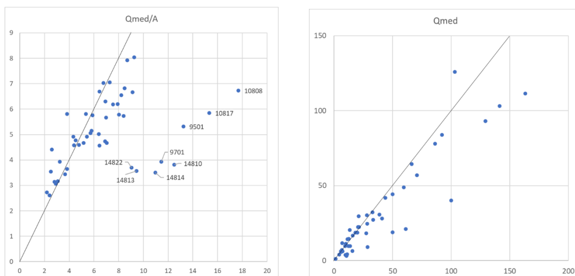
Figura 41. Caudales medios específicos (izquierda) y totales (derecha) observados (eje X) y simulados (eje Y). Fuente: IHCantabria, 2024.
