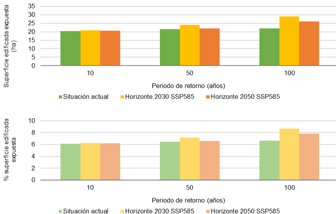
Figura 75. Superficie edificada expuesta (ha) para cada periodo de retorno y escenario climático. Los valores relativos se calculan respecto del total inventariado. Fuente: IHCantabria, 2024.
