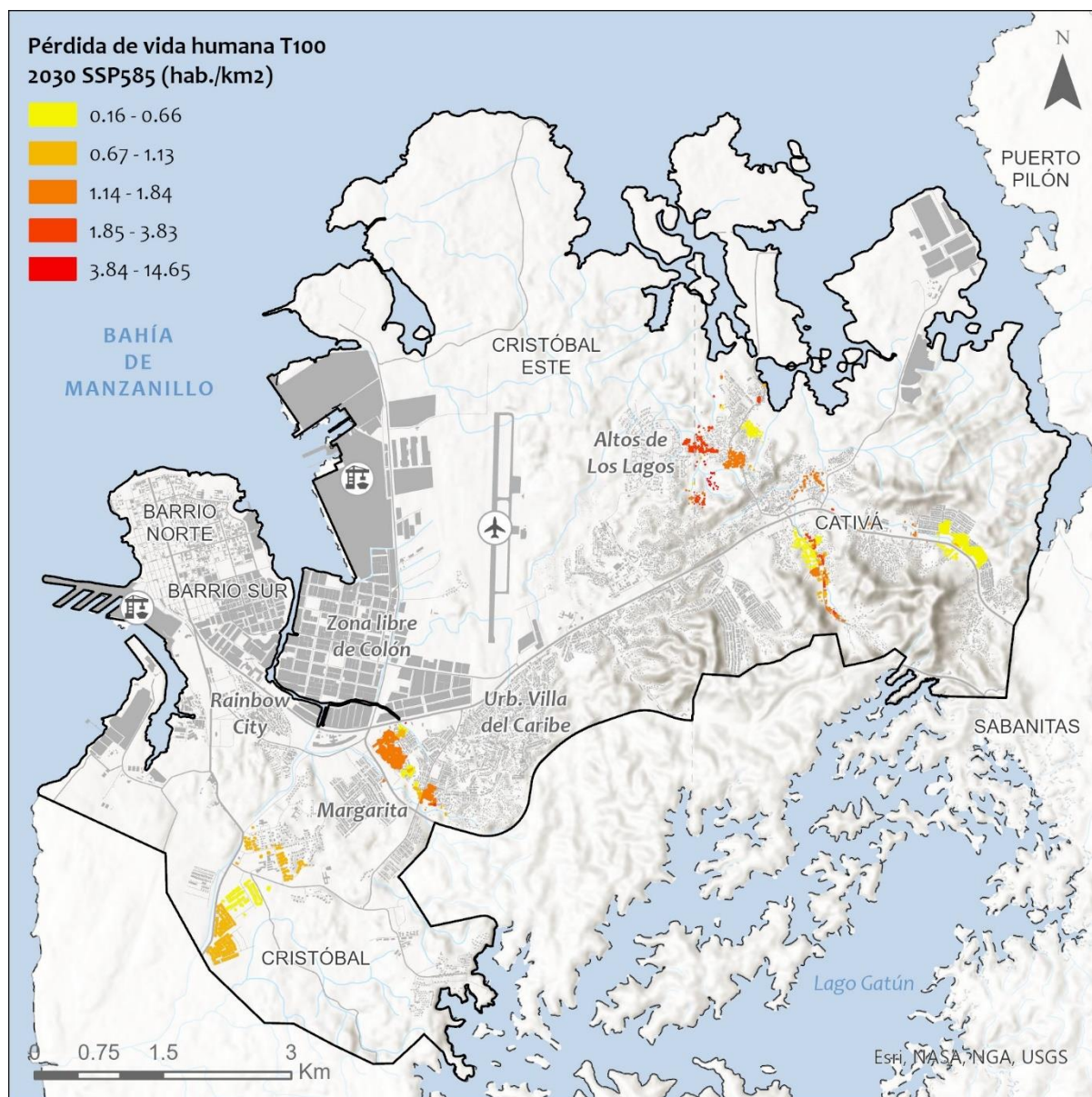
Figura 102. Distribución geográfica de la pérdida de vidas humanas (hab./km2) para 100 años de periodo de retorno en el horizonte 2030 SSP585. Fuente: IHCantabria, 2024.
