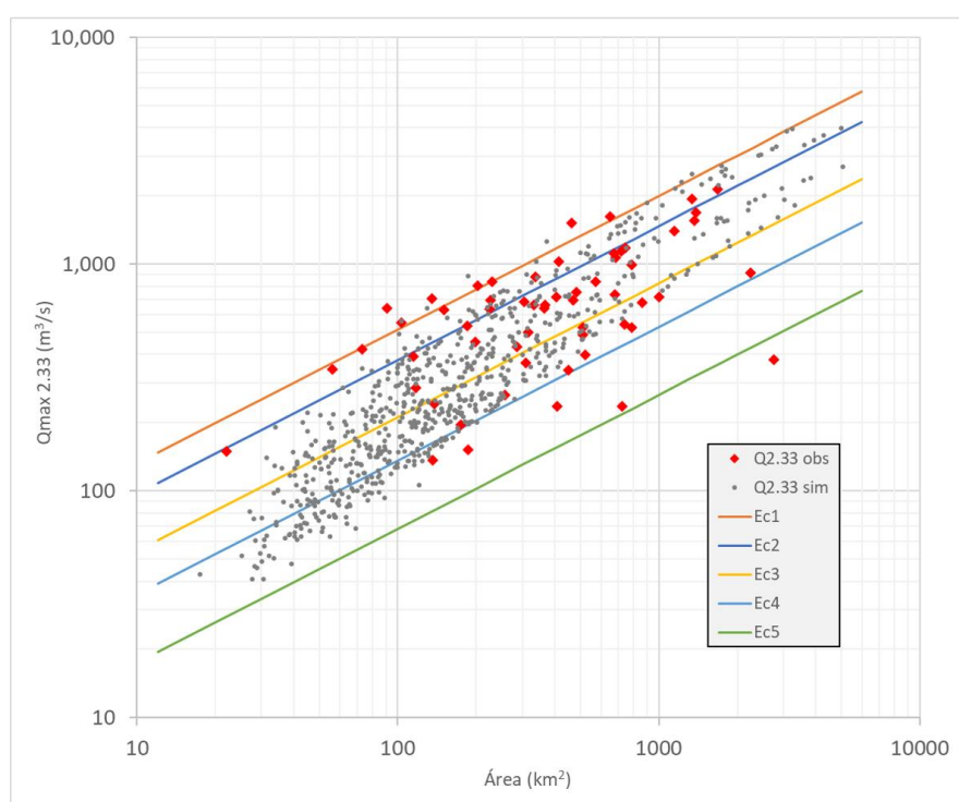
Figura 42. Comparación de caudales Q2.33 observados, simulados, y los ajustes del régimen extremal disponibles por fachadas. Fuente: IHCantabria, 2024.
