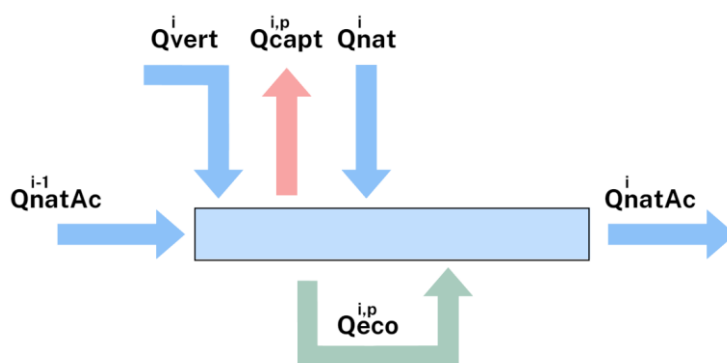
Figura 49. Esquema de funcionamiento del modelo de gestión del agua. Fuente: IHCantabria, 2024.
