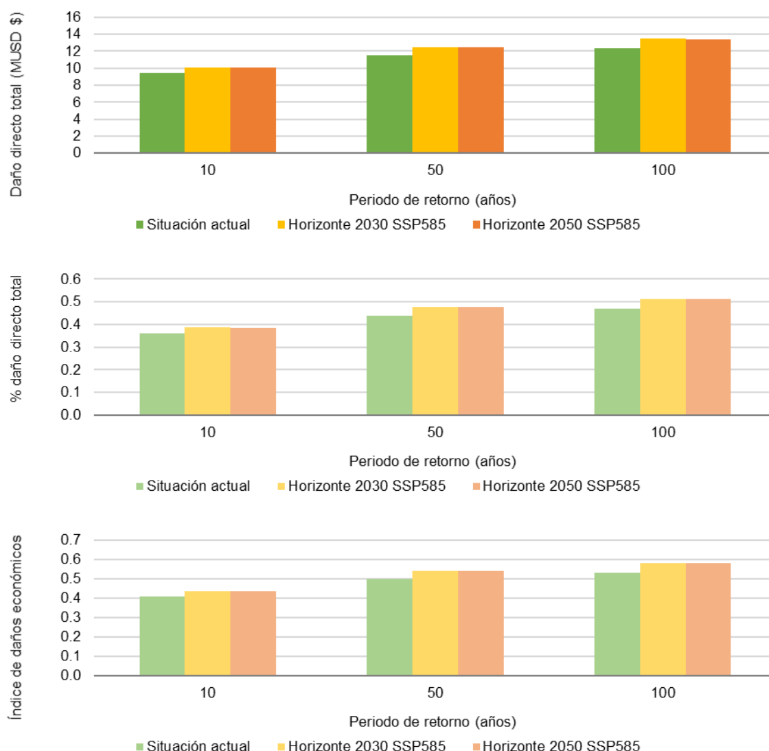
Figura 99. Comparación de resultados de daño económico en los escenarios climáticos considerados, para toda el área de estudio. Fuente: IHCantabria, 2024.
