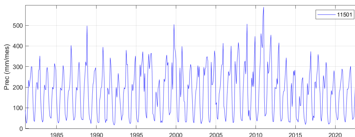
Figura 46. Serie mensual de precipitación (mm/mes) en los lagos Gatún y Alhajuela (subcuenca 11501) para la situación actual. Fuente: IHCantabria, 2024.
