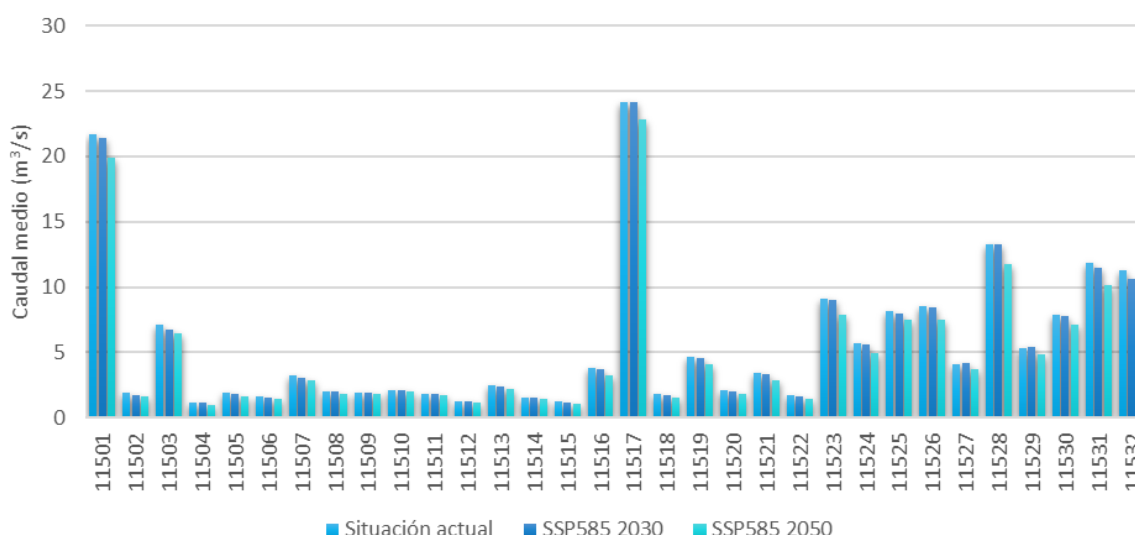
Figura 44. Caudal medio (m³/s) en las subcuencas consideradas para la situación actual y para los escenarios de cambio climático SSP 585 2030 y 2050. Fuente: IHCantabria, 2024.
