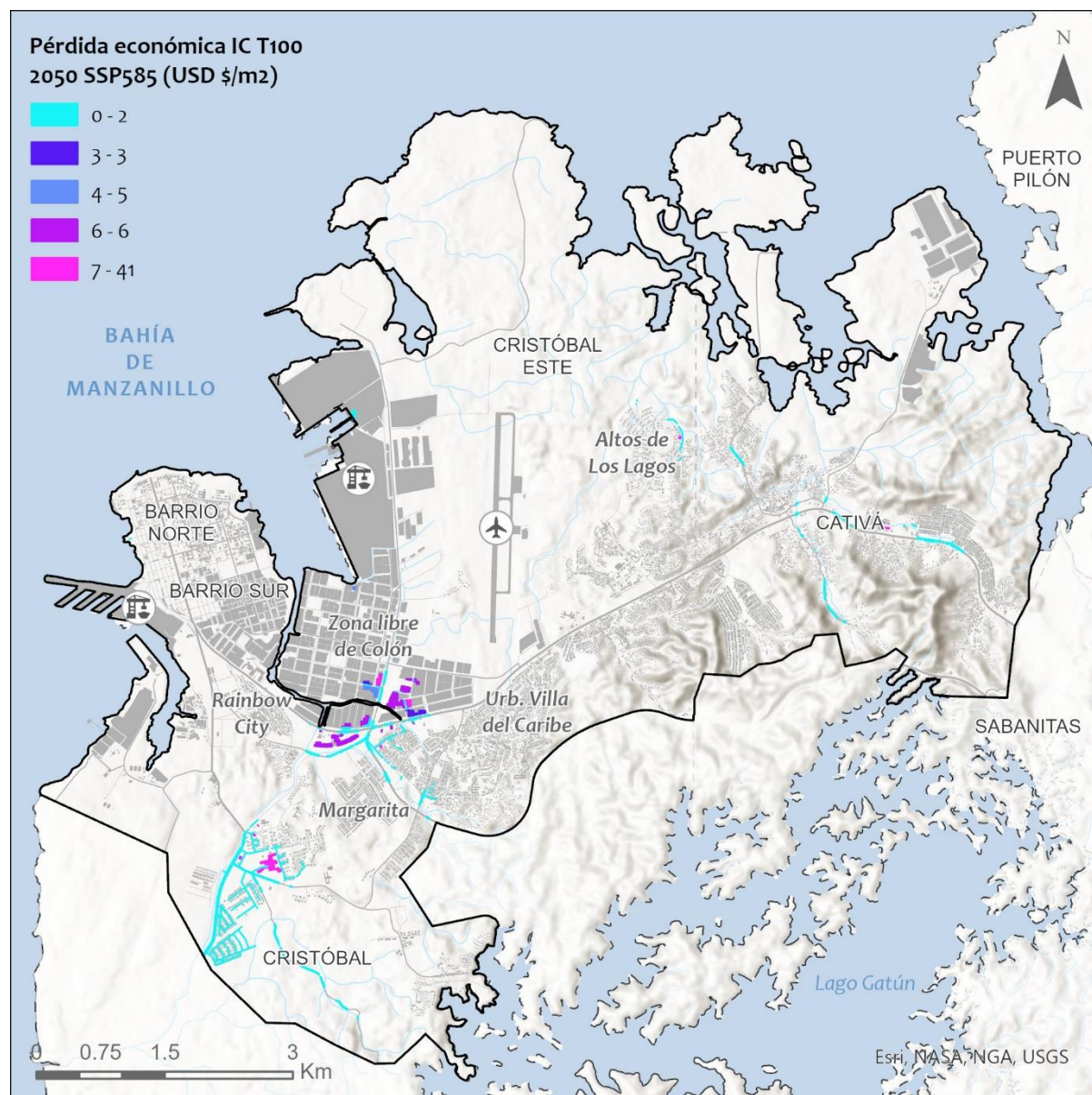
Figura 97. Distribución geográfica de la pérdida económica en IC para 100 años de periodo de retorno (USD $/m 2 ) en el horizonte 2050 SSP585. Fuente: IHCantabria, 2024.
