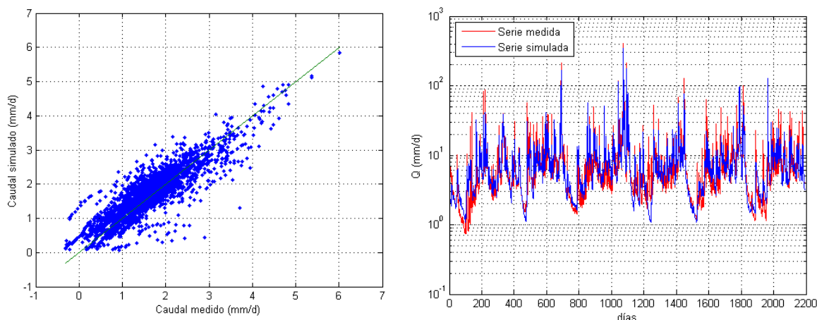
Figura 31. Comparación de caudales diarios medidos y simulados en escala logarítmica (izquierda) y caudales medidos vs. simulados en escala semilogarítmica (derecha) en la estación Peluca. Fuente: IHCantabria, 2015.
