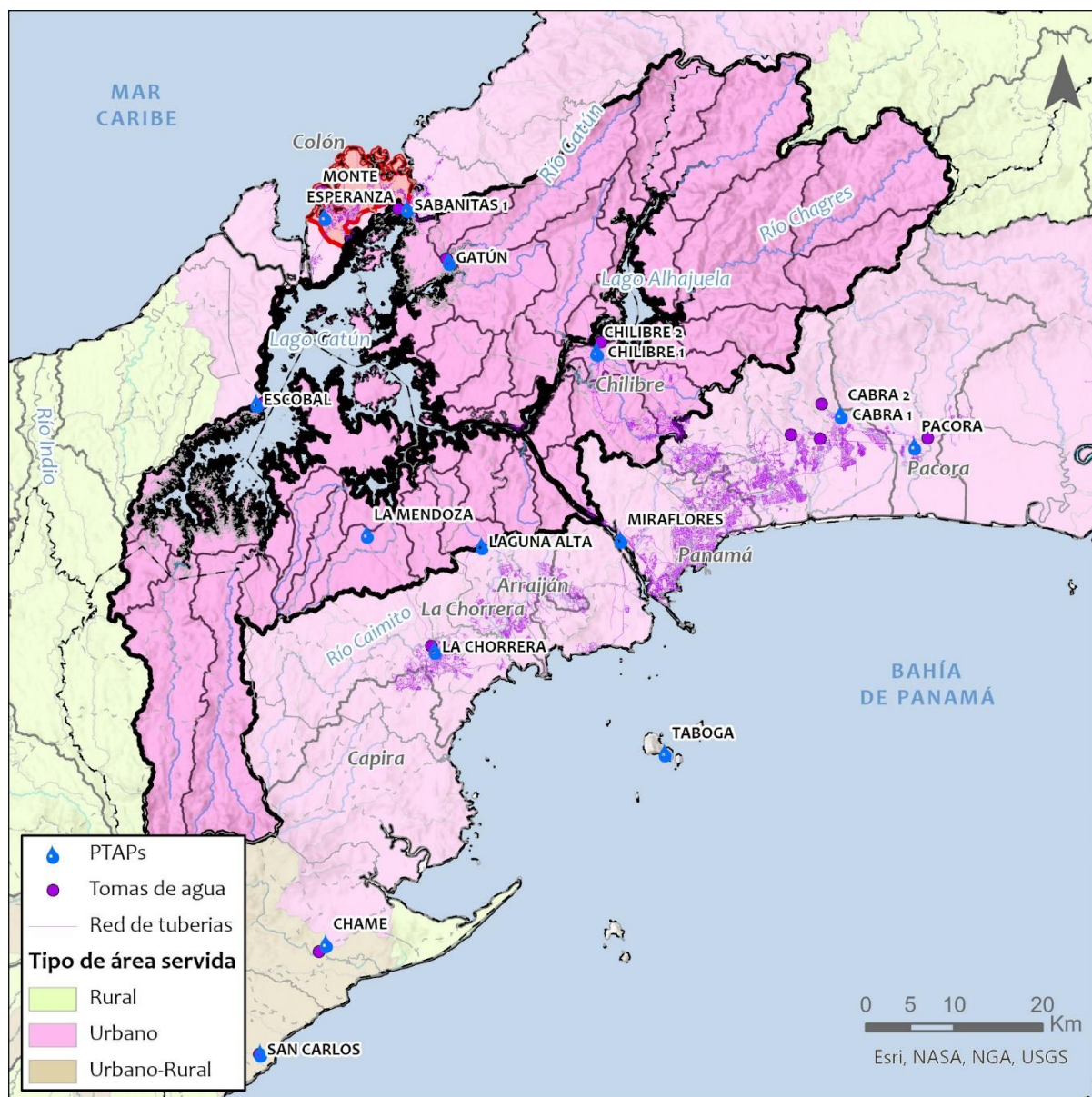
Figura 50. Localización de las plantas potabilizadoras, tomas de agua, red de tuberías y tipo de área servida Fuente: IHCantabria, 2024.
