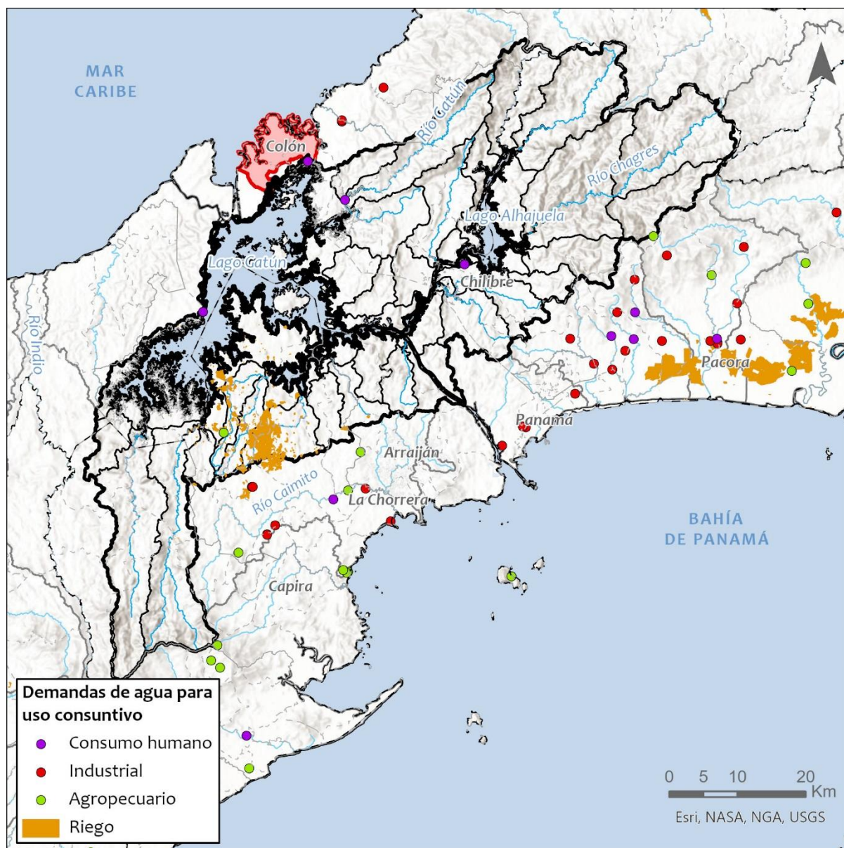
Figura 51. Localización de las demandas de agua en la cuenca del Canal de Panamá. Fuente: IHCantabria, 2024.
