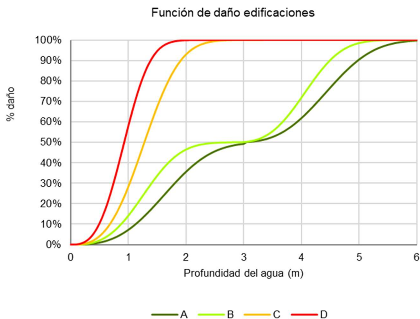
Figura 65. Funciones de daño para calcular los riesgos de inundación. Fuente: IHCantabria, 2024.
