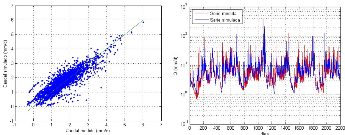
Figura 28. Comparación de caudales diarios medidos y simulados en escala logarítmica (izquierda) y caudales medidos vs. simulados en escala semilogarítmica (derecha) en la estación Peluca. Fuente: IHCantabria, 2015.
