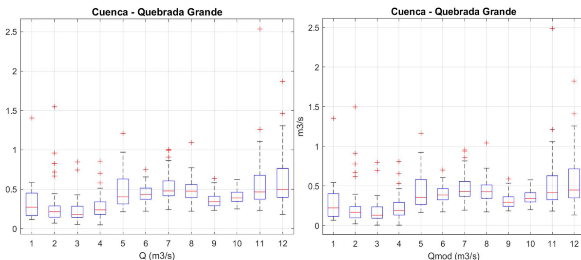
Figura 48. Boxplot de caudales naturales y modificados ( m^3/s ) en la cuenca del Big Creek, para la situación actual. Fuente: IHCantabria, 2024.
