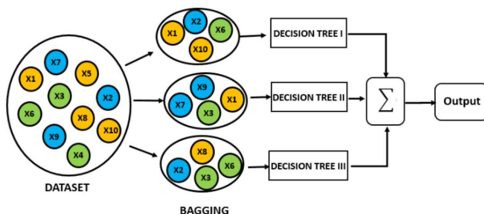
Figura 11. Esquema resumen de algoritmo RF y proceso bagging . Fuente: (Espinosa-Zuñiga, 2020).
