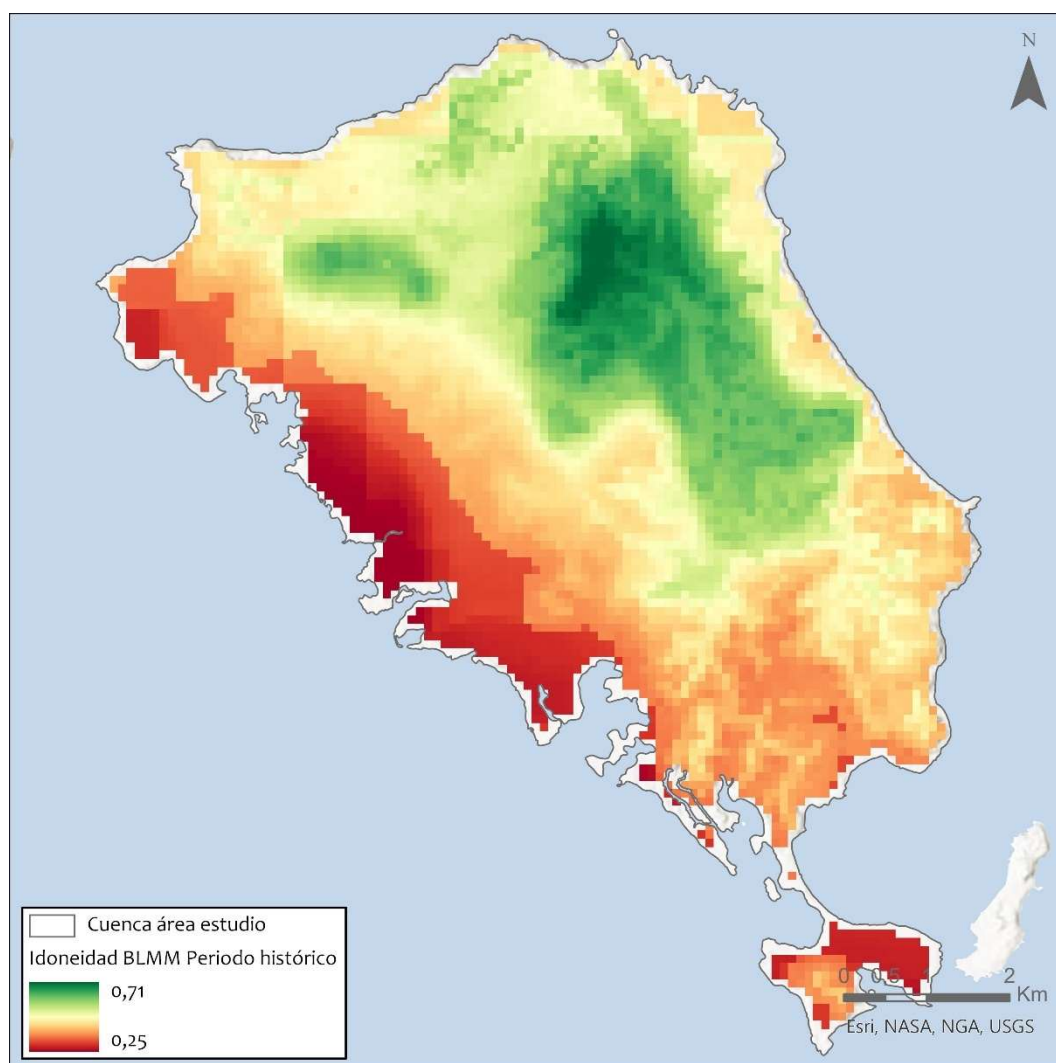
Figura 12. Mapa de idoneidad del bosque latifoliado mixto maduro para la situación actual para la cuenca drenante de Isla Colón, Bocas del Toro. Fuente: IHCantabria, 2024.
