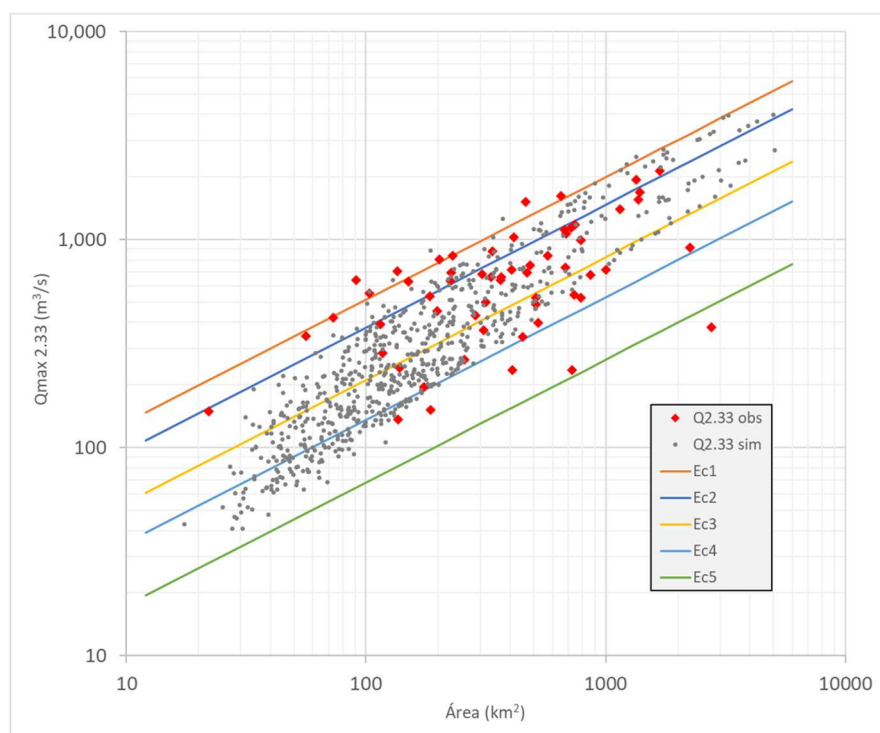
Figura 39. Comparación de caudales Q2.33 observados, simulados, y los ajustes del régimen extremal disponibles por fachadas. Fuente: IHCantabria, 2024.
