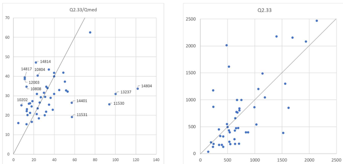
Figura 40. Caudales Q2.33 específicos (izquierda) y totales (derecha) observados (eje X) y simulados (eje Y). Fuente: IHCantabria, 2024.
